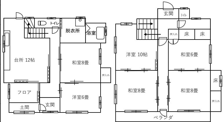
【間取り】
