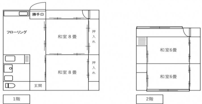
【間取り図】
